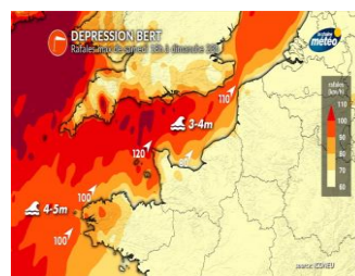
Alerte Météo France pour la tempête Bret
